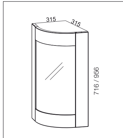
■ Íves üvegajtó keret
